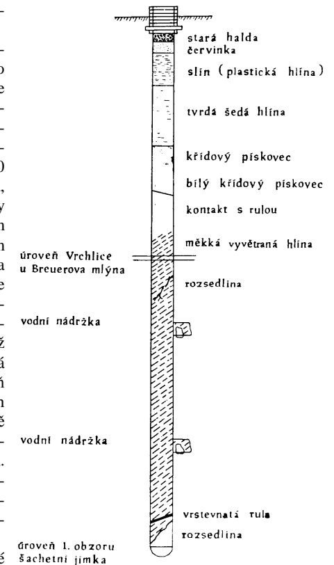
Průřez kutací šachty na Rovinách
